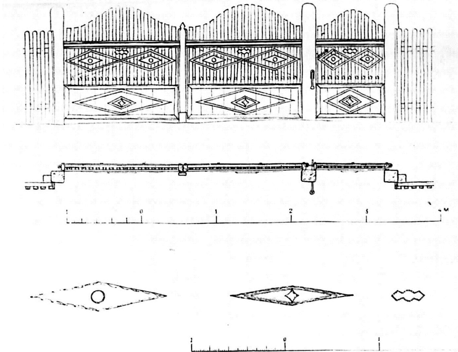
Poartă de lemn cu ornamente geometrice. Schiță grafică. Cercetări etnografice de teren. ASCASM 1975. Fondul 24, inv. 18, f.51.
