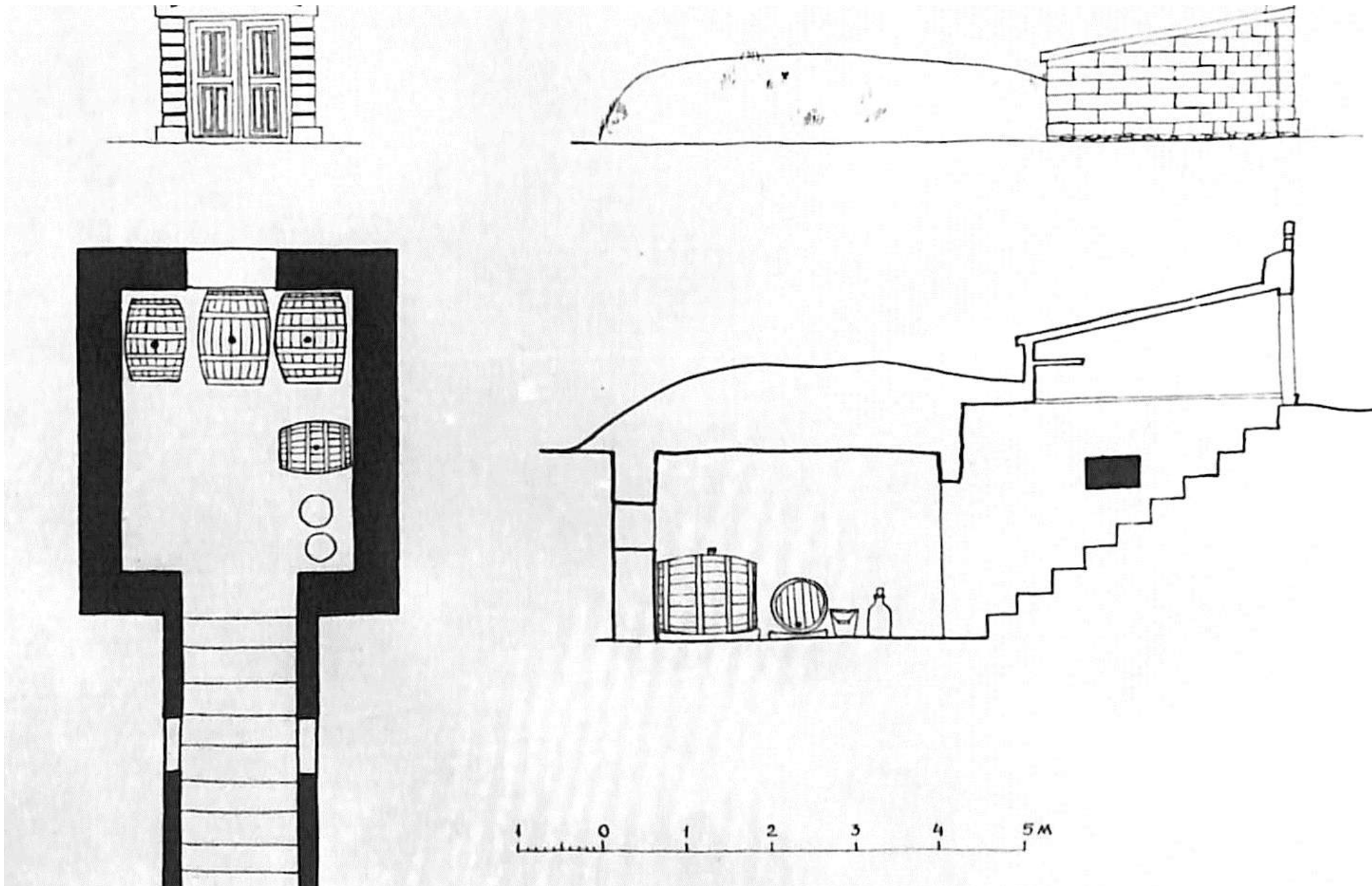
Beci. Schiță grafică. Cercetări etnografice de teren. ASCASM 1975. Fondul 24, d.18, f.37.
