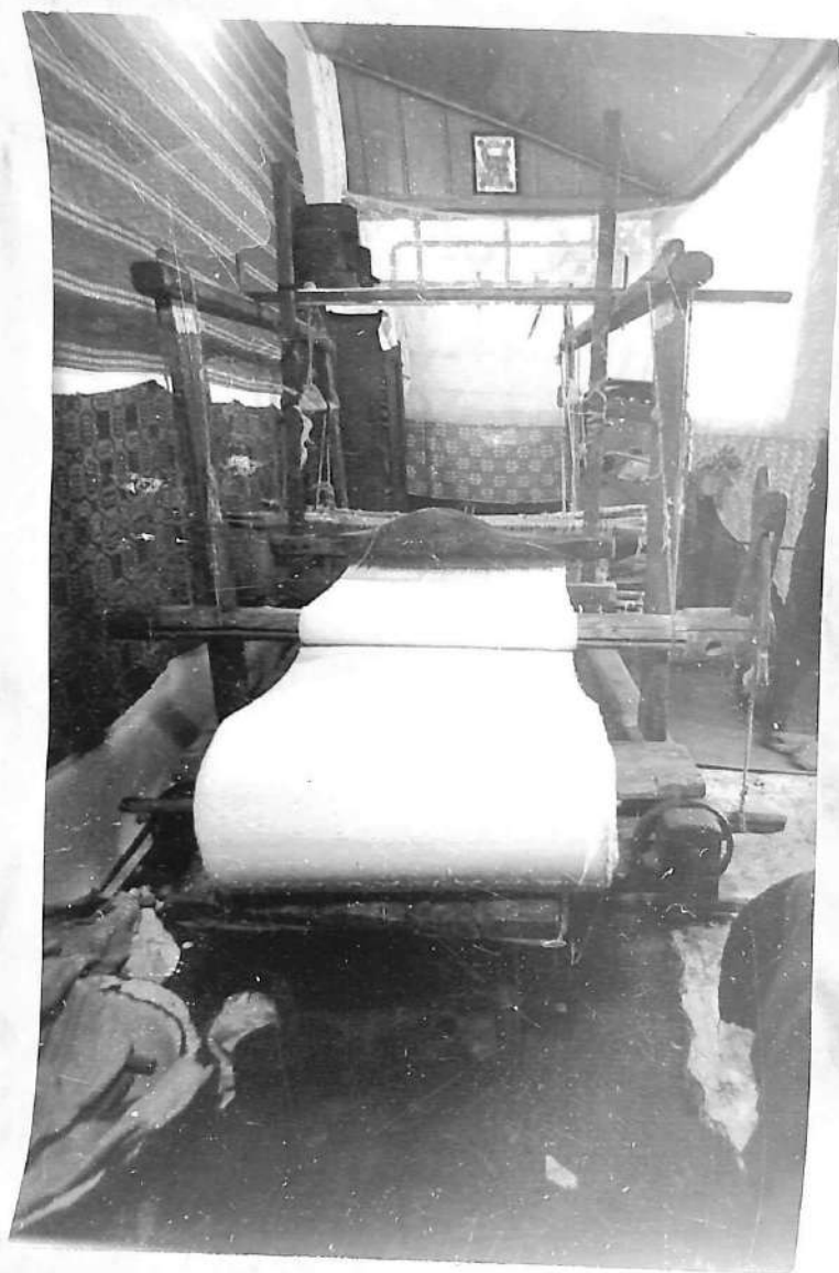
Тканье халата на горизонтальном ткацком стане
